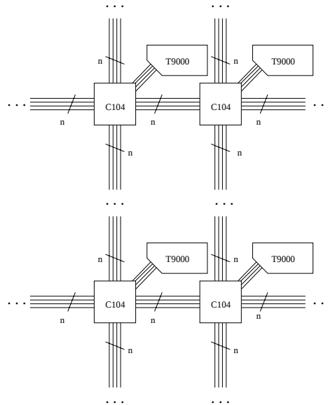
Figura 3: Una red basada en el transputer T9000 y el encaminador C104
