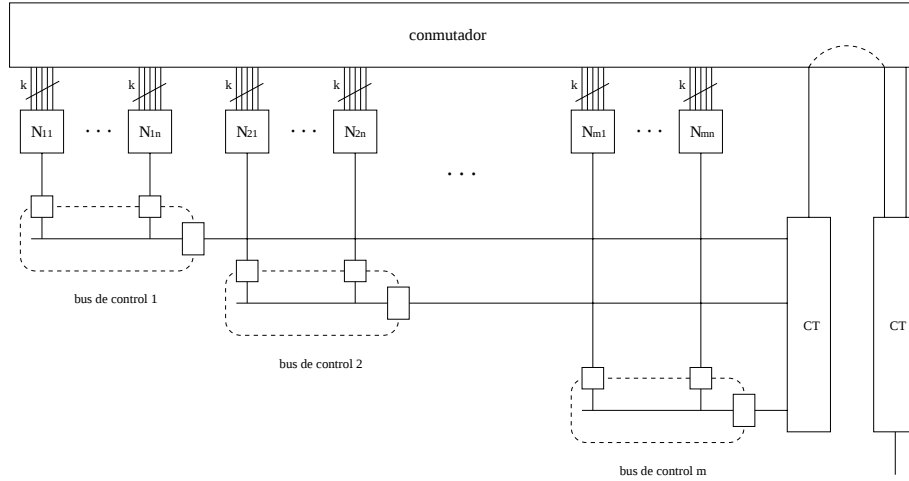
Figura 5: Estructura general de una arquitectura reconfigurable basada en bus serie
