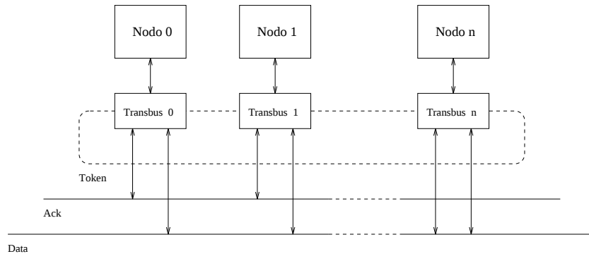
Figura 6: Interconexión de los nodos mediante el controlador TRANSBUS
