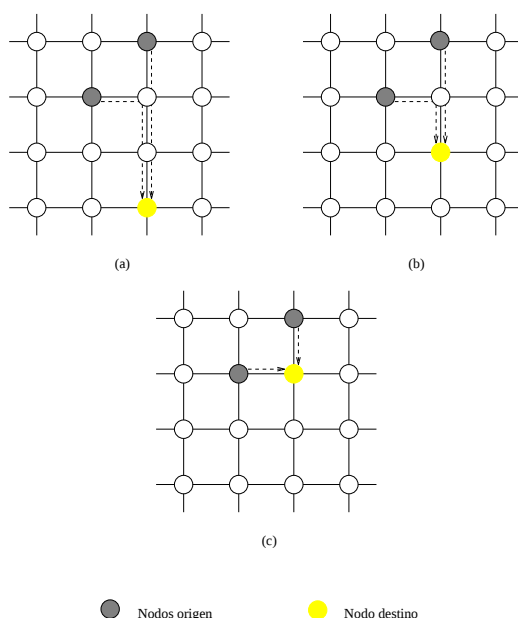
Figura 1: Ejemplo de los efectos del algoritmo de reconfiguración
