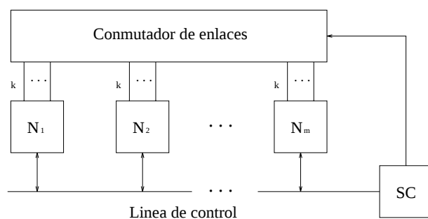
Figura 4: Estructura del sistema para la reconfiguración dinámica
